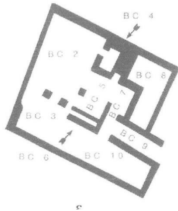
Εικόνα 16. Κάτοψη του Building of the Pillar Partitions.
