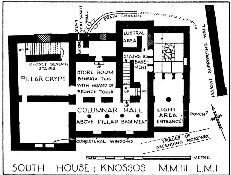
Εικόνα 3. Κάτοψη Νότιας Οικία/South House.
